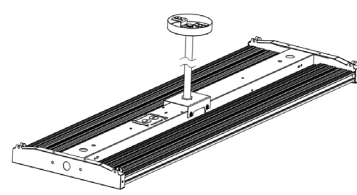
LLHB4-RODKIT
